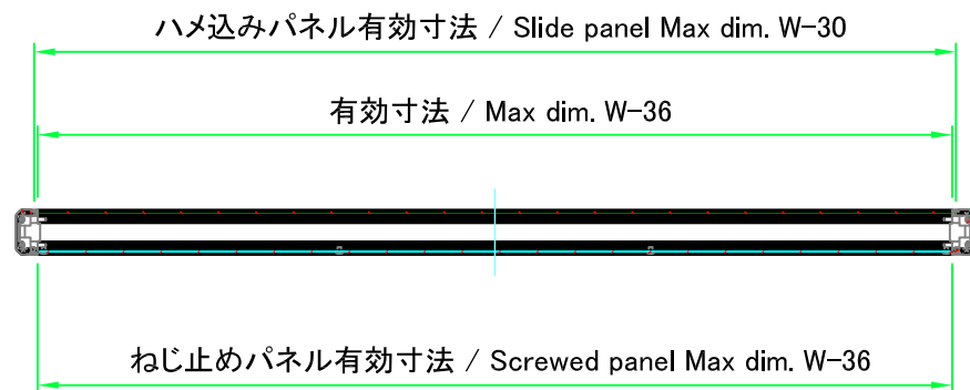
A-A (1:7)
